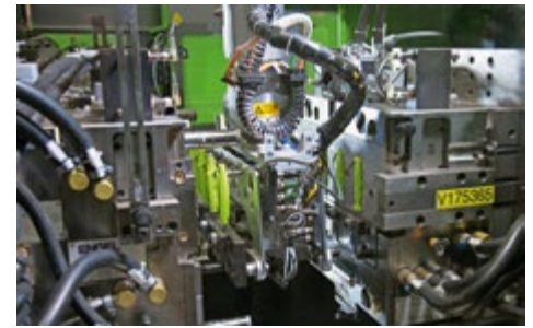
Viper Linearroboter übernehmen das Platzieren der Klingen und Vorspritzlinge sowie das Entformen. Derselbe Viper, der die Klingen ins Werkzeug einlegt, entnimmt die Vorspritzlinge.
